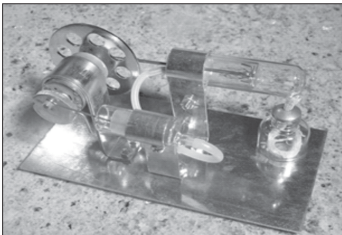
Silnik Stirlinga
