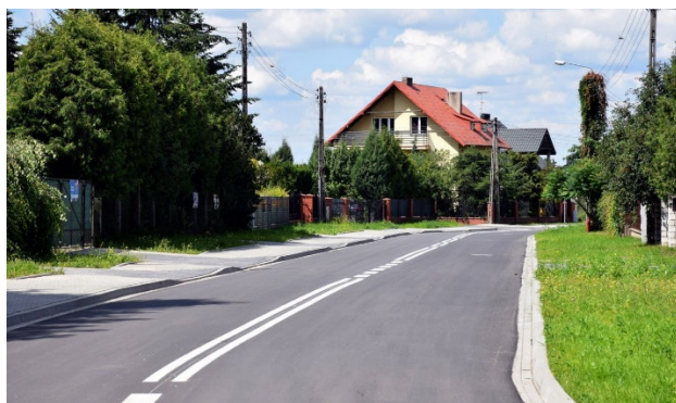
Fot. Przebudowa ul. Orlej
